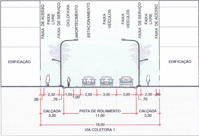
Figura 6-12: Seção da via coletora tipo 1
