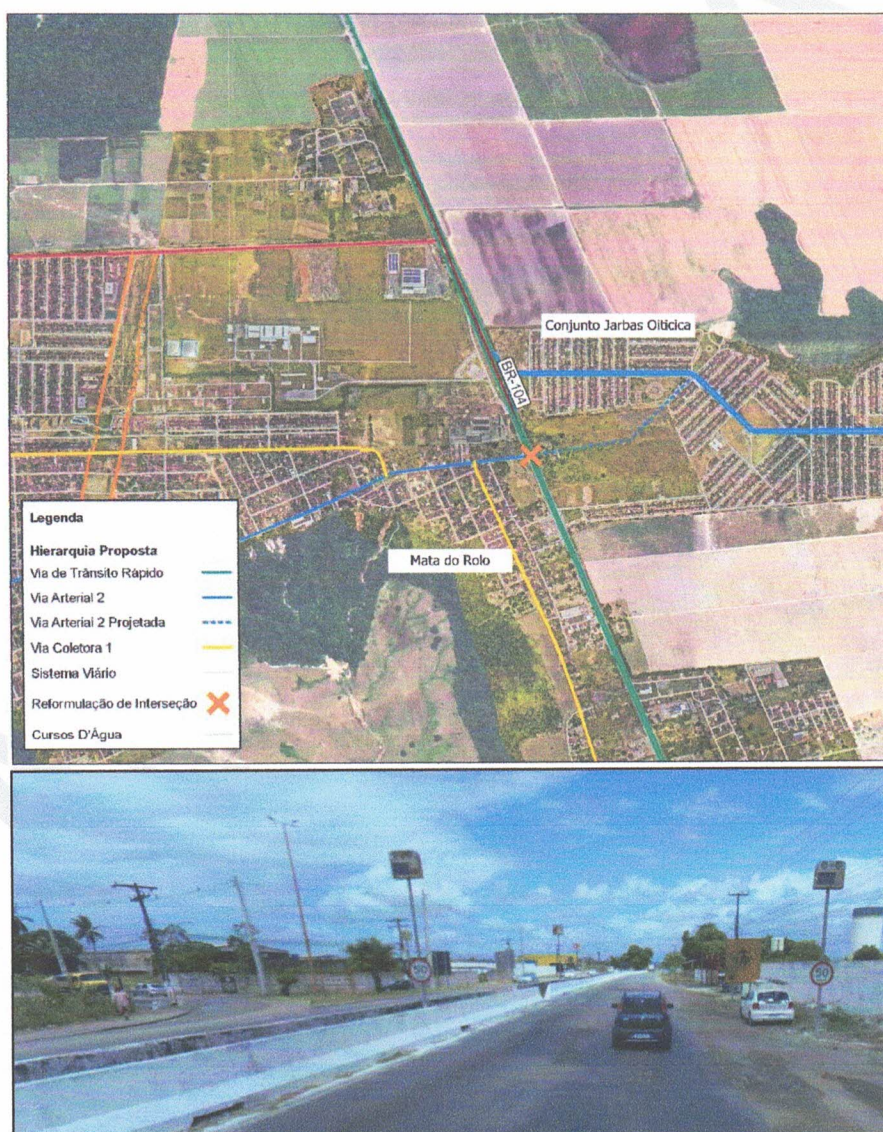
Figura 6-18: Proposta de interseção em desnível com rotatória e trincheira em Rio Largo
