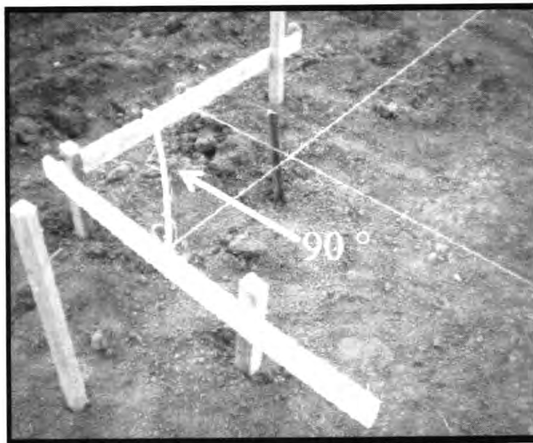
Esquadro da locação
