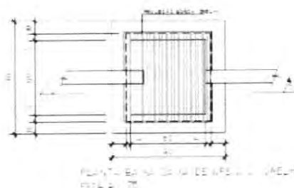
DETALHE CAIXA DE ÁREA E ESGOTO PLUVIAL 60X60CM
